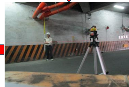
⑤ 施工現場放樣出水口放樣
